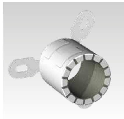
Brandrohrmanschette Rorcol AV60 für Alu-Verbundrohre
